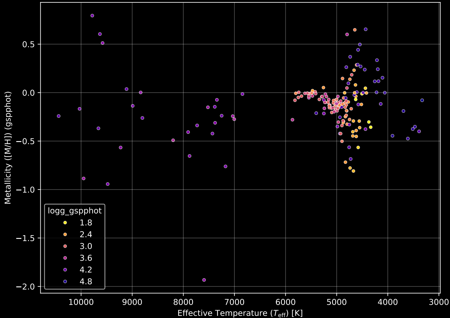
APOGEE DR17 Field: [173+18] Stellar Population Parameters (n= 181)
